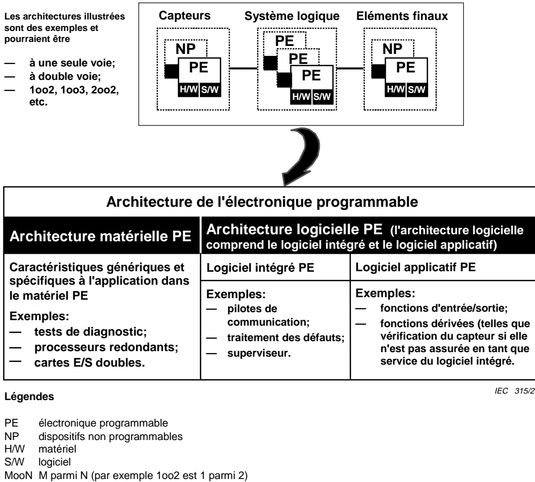
Figure 4 – Relation entre l'architecture matérielle et l'architecture logicielle de l'électronique programmable
